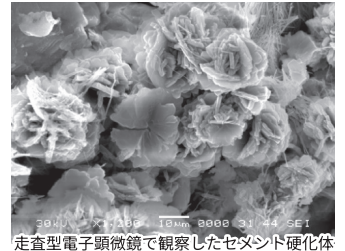
走査型電子顕微鏡で観察したセメント硬化体
